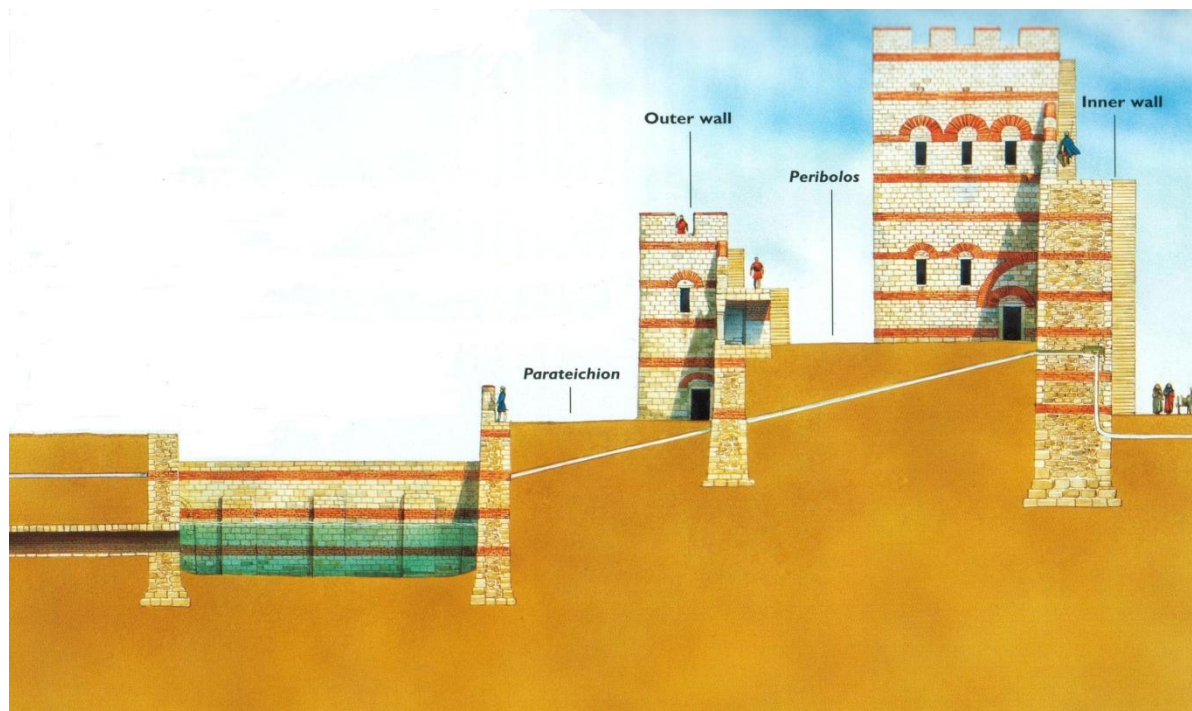
(Σκαρίφημα του τριπλού τείχους της Κωνσταντινούπολης και της τάφρου, S. Turnbull, Walls of Constantinople , Osprey Publishing, 2004).
